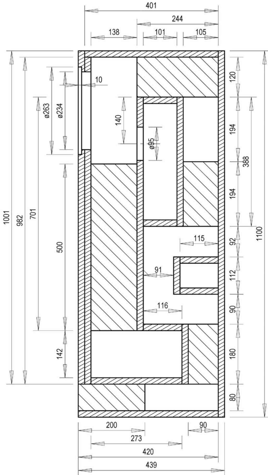
Zyklop-Sub II aus HOBBY HiFi 5/2016 mit Anpassung
